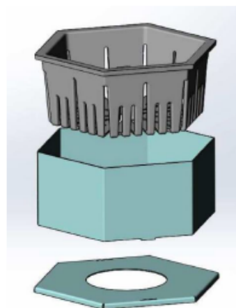
Q7 HEX avec plaque hexagonale
